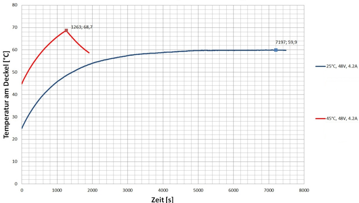
PD4-E Temperaturmessung
