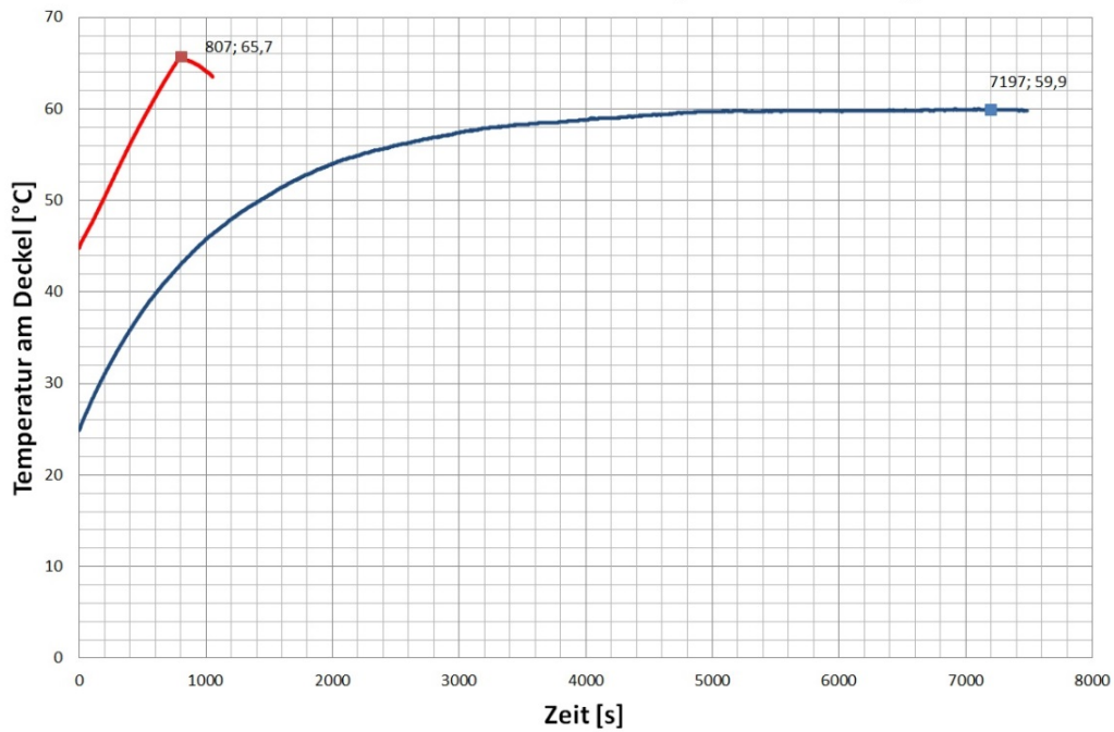
PD4-EB59CD Temperaturmessung
