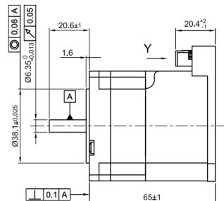
Seitenansicht
