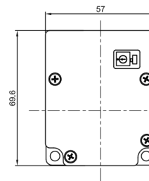
Rückansicht
