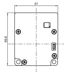
Rückansicht
