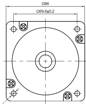
Frontansicht und Montierung
