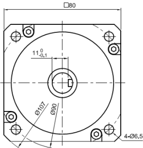
Frontansicht und Montierung
