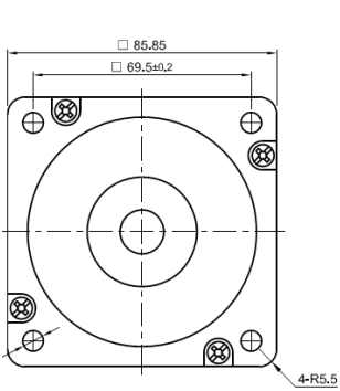
Frontansicht und Montierung
