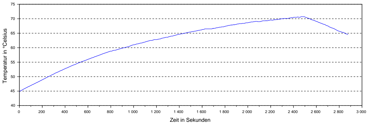
PD6-CB87: Steuerungstemperatur bei 45° Celsius Umgebungstemperatur und 6.5A Motorstrom
