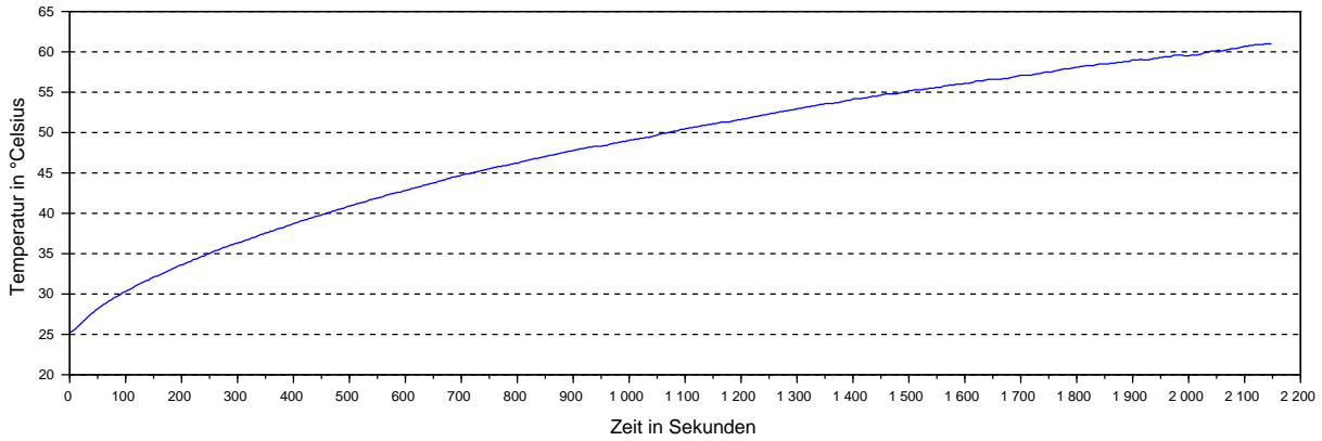
PD6-C: Steuerungstemperatur bei 25° Celsius Umgebungstemperatur und 9.5A Motorstrom
