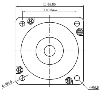
Frontansicht und Montierung
