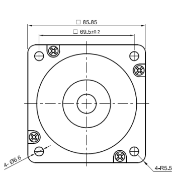
Frontansicht und Montierung
