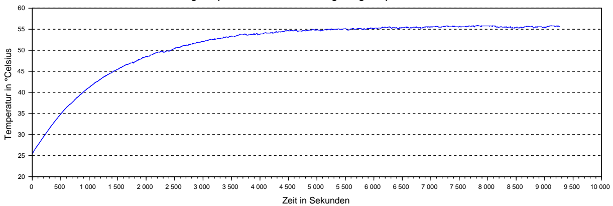
PD6-CB87: Steuerungstemperatur bei 25° Celsius Umgebungstemperatur und 6.5A Motorstrom
