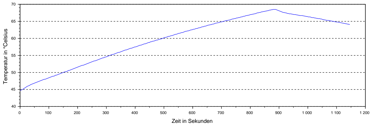
PD6-CB80: Steuerungstemperatur bei 45° Celsius Umgebungstemperatur und 14A Motorstrom
