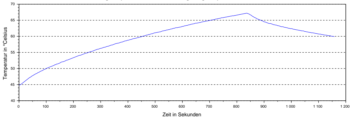
PD6-C: Steuerungstemperatur bei 45° Celsius Umgebungstemperatur und 9.5A Motorstrom
