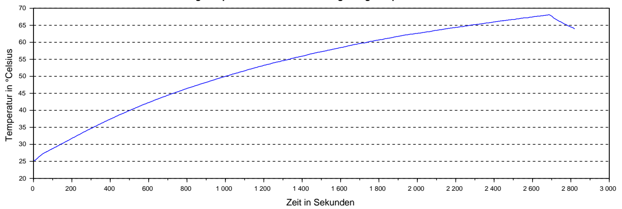
PD6-CB80: Steuerungstemperatur bei 25° Celsius Umgebungstemperatur und 14A Motorstrom
