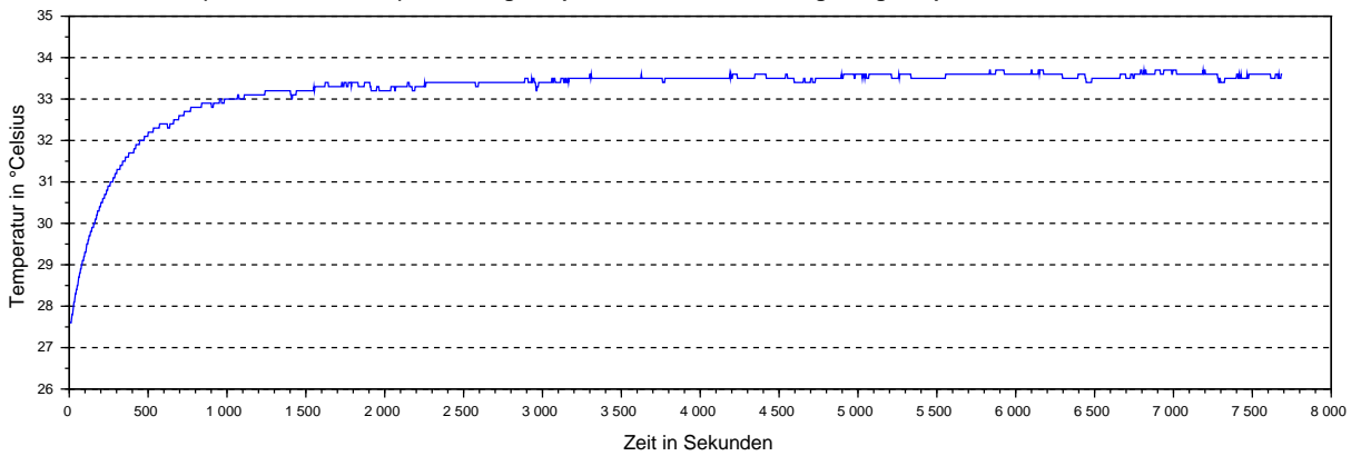
C5-E (Low current version): Steuerungstemperatur bei 25° Celsius Umgebungstemperatur und 6A Motorstrom
