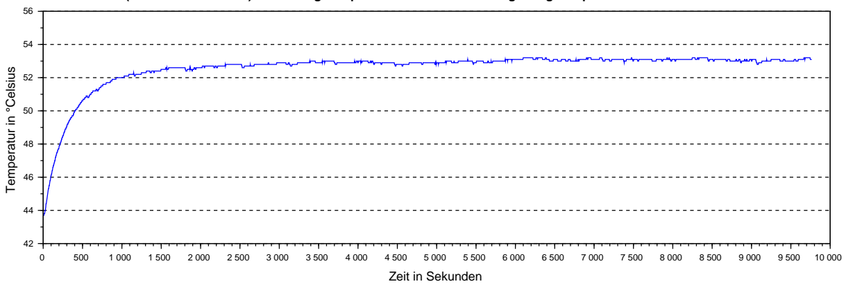
C5-E (Low current version): Steuerungstemperatur bei 45° Celsius Umgebungstemperatur und 6A Motorstrom
