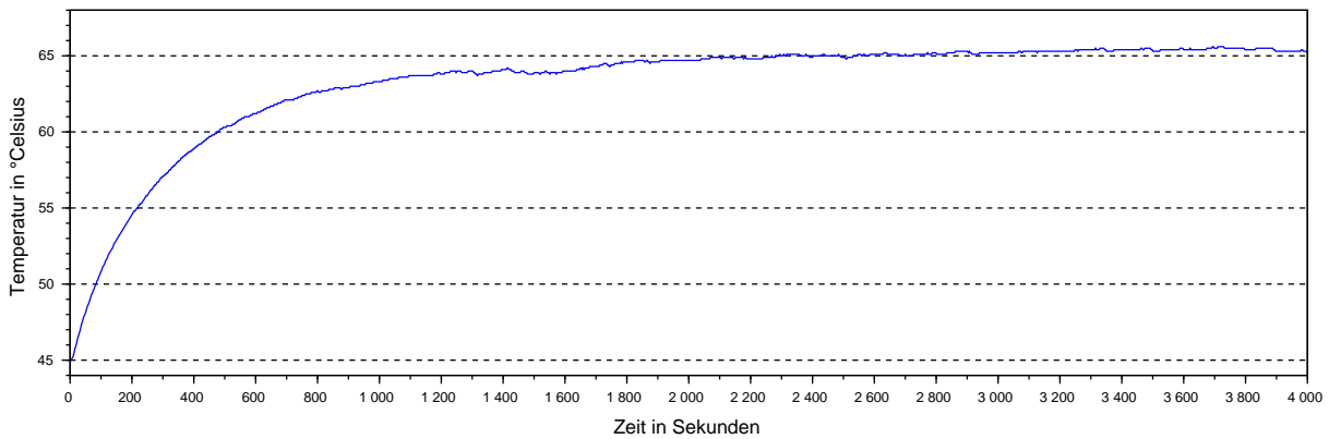
C5: Steuerungstemperatur bei 45° Celsius Umgebungstemperatur und 6A Motorstrom
