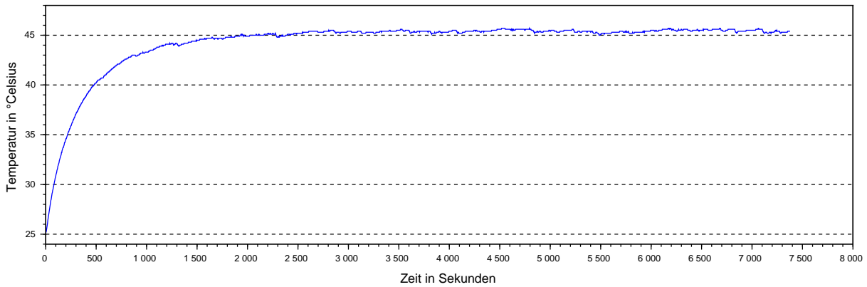
C5: Steuerungstemperatur bei 25° Celsius Umgebungstemperatur und 6A Motorstrom
