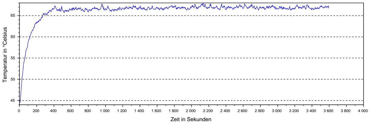
CL3-E: Steuerungstemperatur bei 25° Celsius Umgebungstemperatur und 3A Motorstrom
