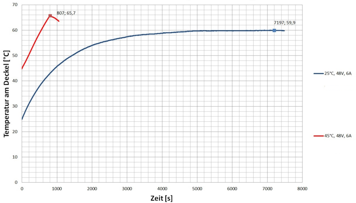
PD4-EB59CD Temperaturmessung
