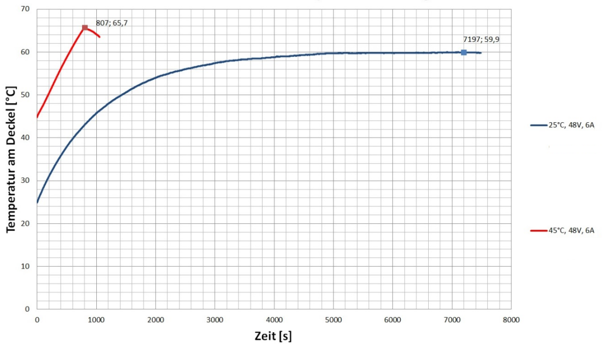
PD4-EB59CD Temperaturmessung
