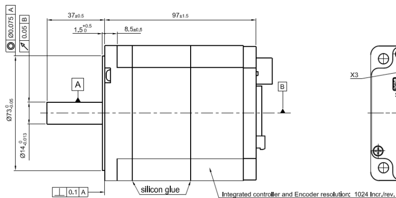
Seitenansicht
